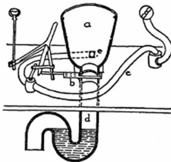
Joonis 7. A. Cummings' vesiklosett a) kauss, b) liugklapp, d) sifoontlõks. (Brown, 2005: 21)
