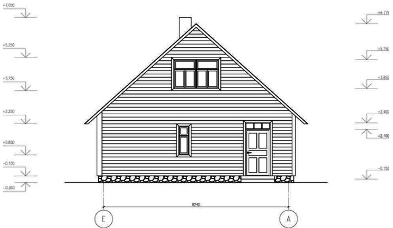
Joonis 4. Talu vaade E-A.
