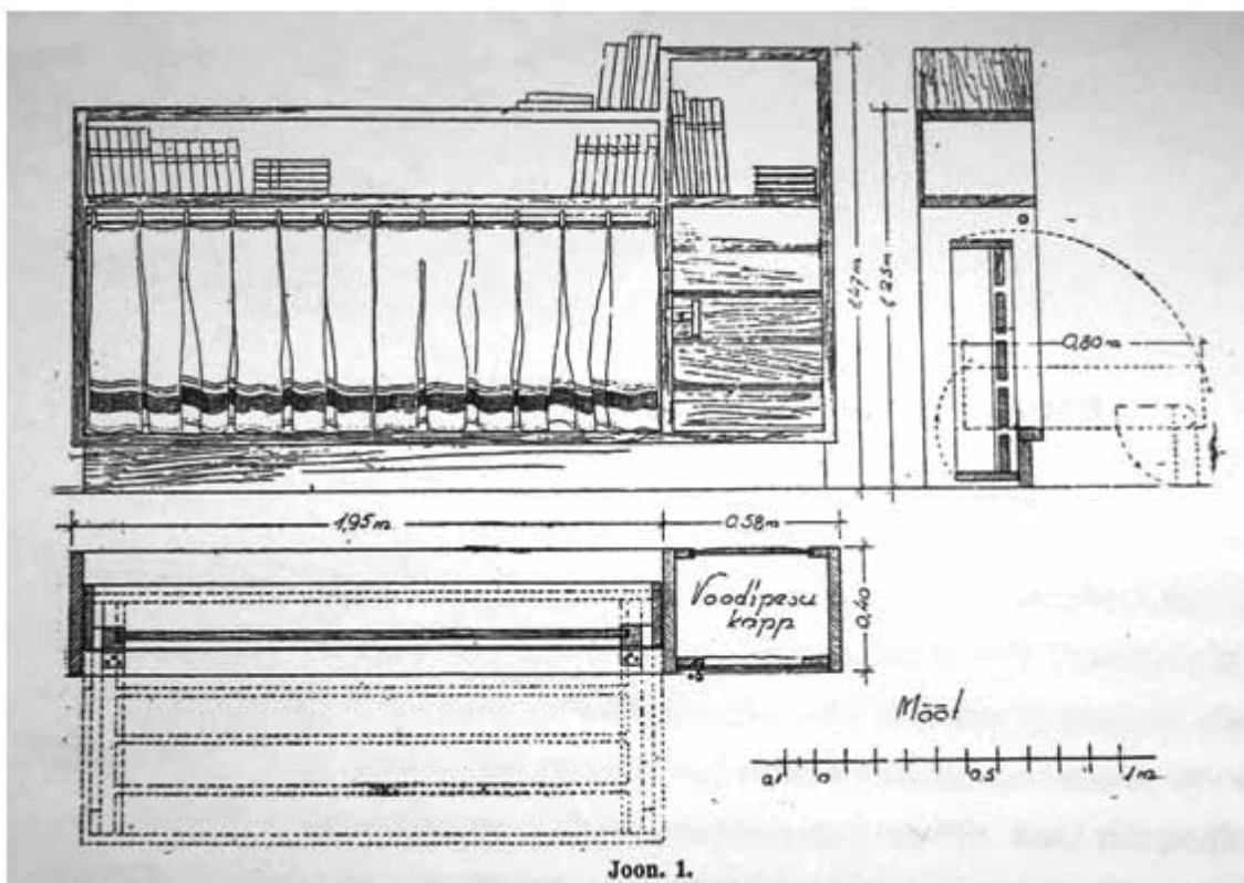
Joonis 9. Magamistoa sisseehitatud mööbli joonis (Kaunis Kodu, 1934: 6).
